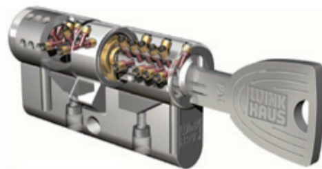
Il cilindro delle nuove serrature Piccioni
